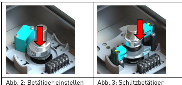
Abb. 2: Betätiger einstellen
