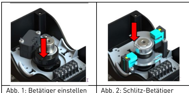
Abb. 1: Betätiger einstellen
